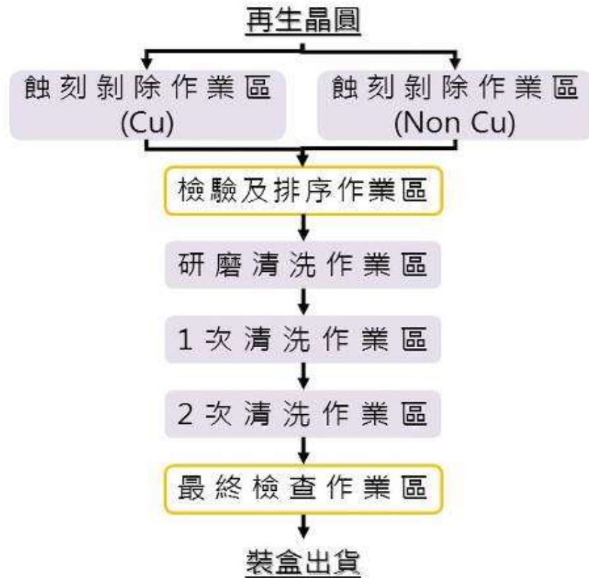
圖 1-3、製程流程圖
