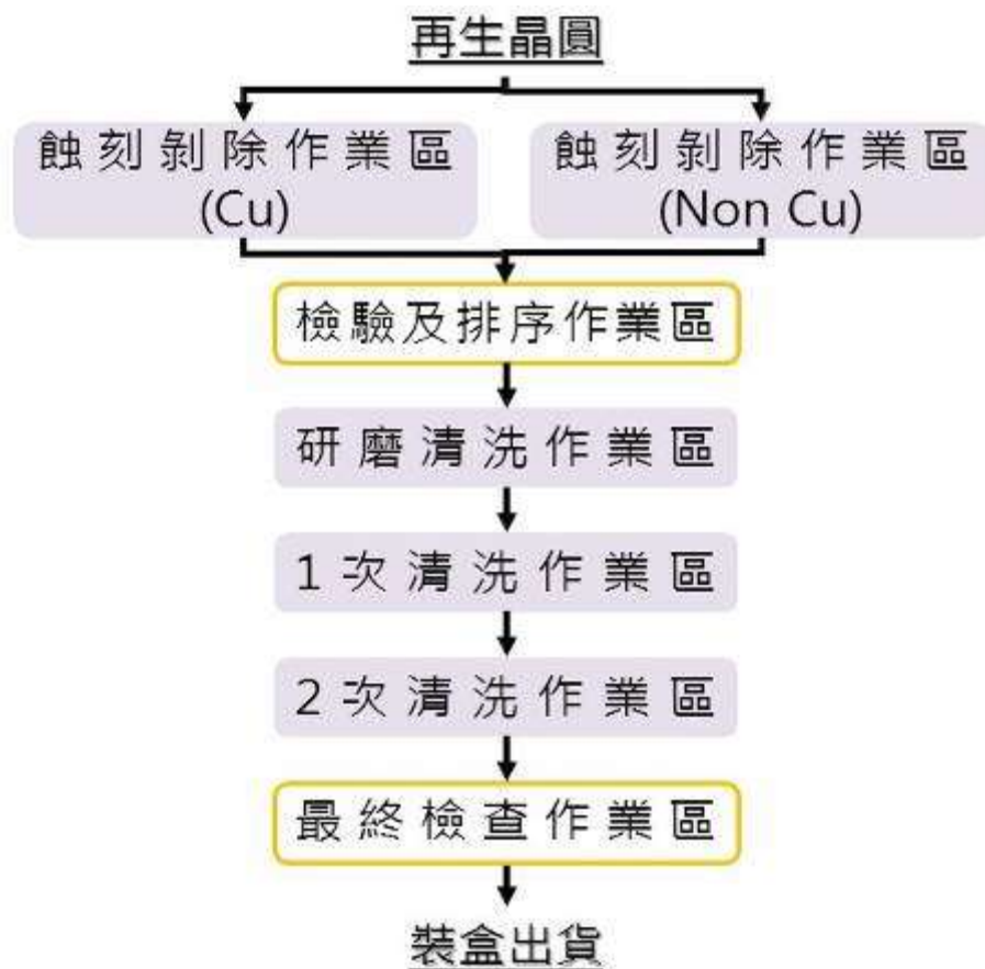
圖 1-3、製程流程圖
